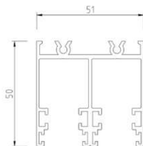
Guida superiore 2 vie
