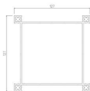
Pilastro 3706 g/ml cod. NB0290
