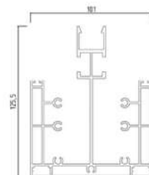
Gronda Centrale 3810 g/ml cod. NB0296
