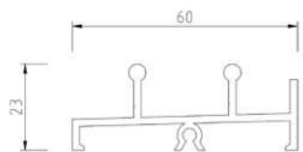
Binario inferiore 2 vie
