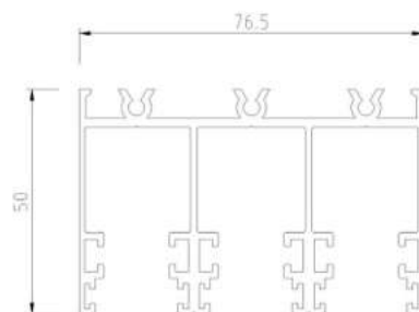
Guida superiore 3 vie
