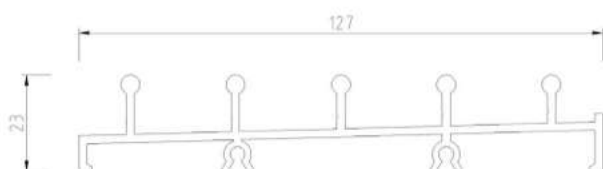
Binario inferiore 5 vie
